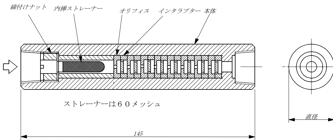
SS型断面図
